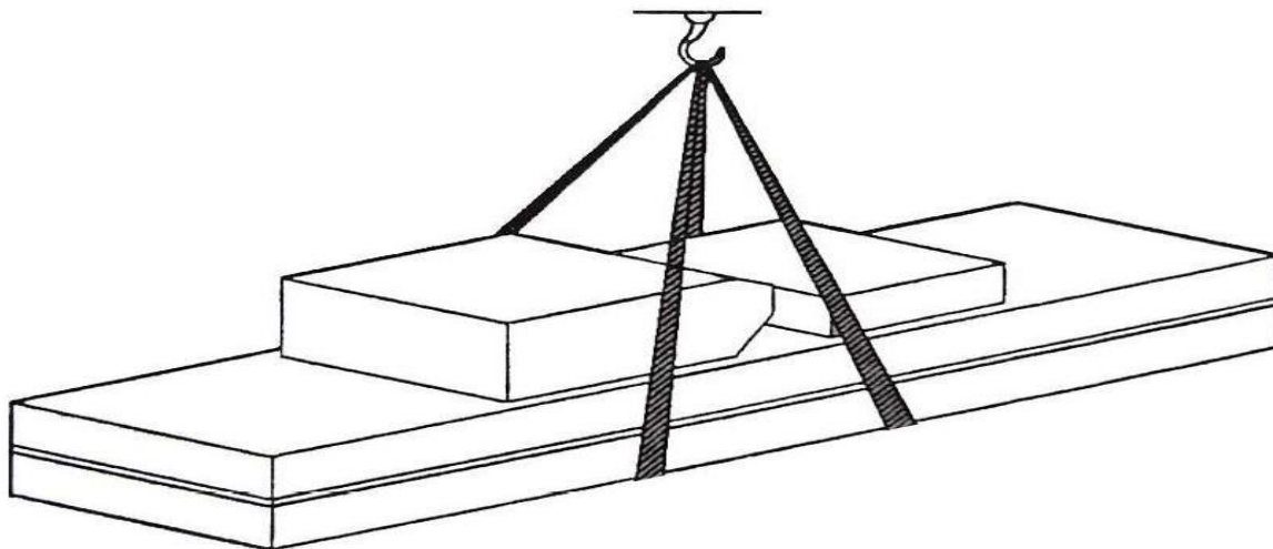
Рис. 1 Стрповка оборудования
