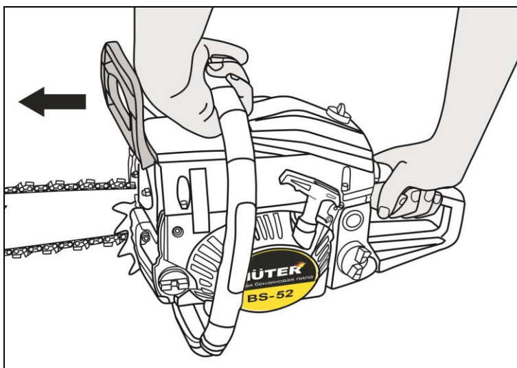
Рис. 22. Остановка цепи тормозом цепи
