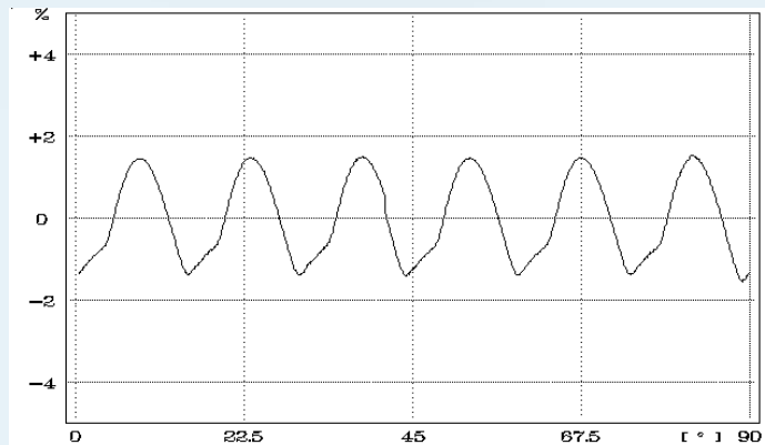
Обрыв обмотки статора
