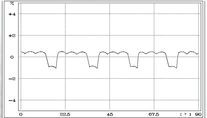
Пробой диода обратной полярности
