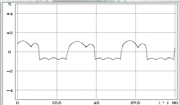
Обрыв диода прямой полярности
