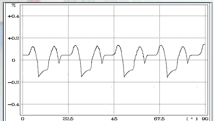
Пробой диода прямой полярности
